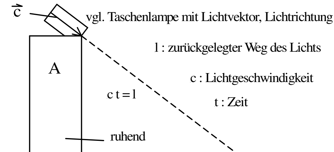
Bild 2: Weg des Lichts unumstritten, zweifellos
